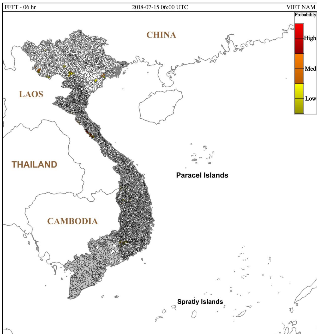
Hình 3: Nguy cơ lũ quét trong 6 giờ tới tại các lưu vực từ 13h ngày 15/7/2018 giờ địa phương
