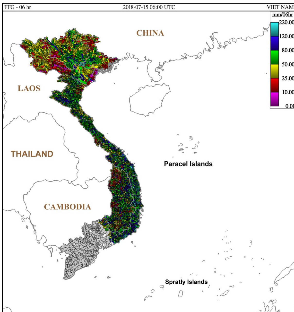
Hình 1. Ngưỡng mưa định hướng có khả năng sinh lũ quét trong 6 giờ tới tại các lưu vực từ 13h ngày 15/7/2018 giờ địa phương
