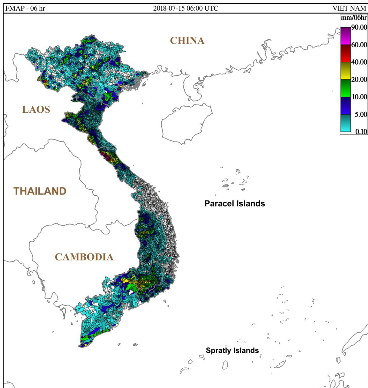
Hình 2: Dự báo lượng mưa trung bình lưu vực 6 giờ tính từ 13h ngày 15/7/2018 giờ địa phương
