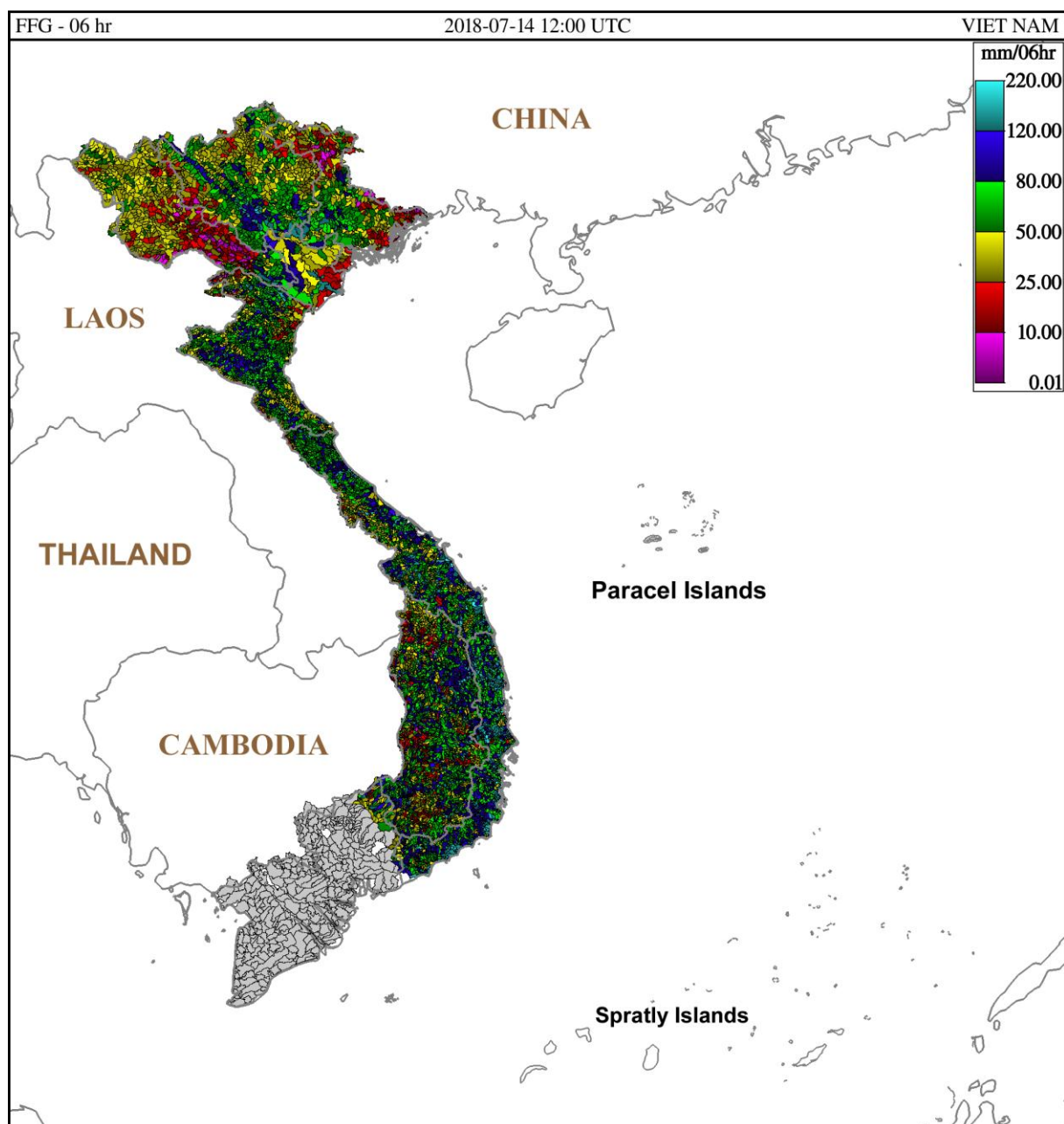
Hình 1. Ngưỡng mưa định hướng có khả năng sinh lũ quét trong 6 giờ tới tại các lưu vực từ 19h ngày 14/07/2018 giờ địa phương
