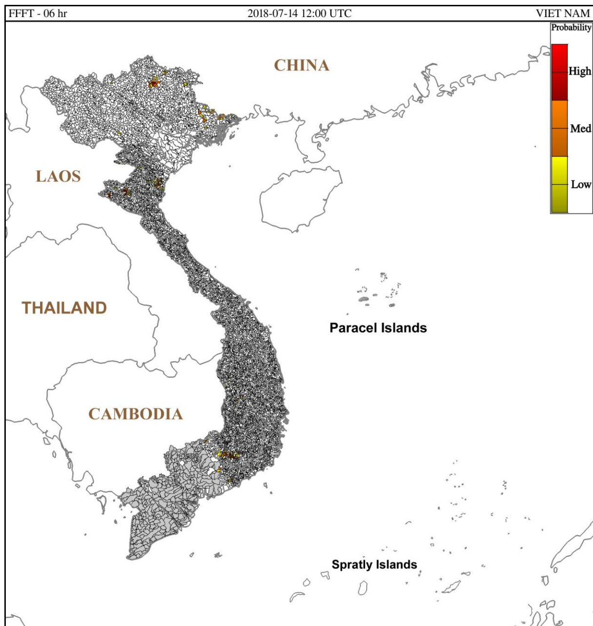
Hình 3: Nguy cơ lũ quét trong 6 giờ tới tại các lưu vực từ 19h ngày 14/07/2018 giờ địa phương
