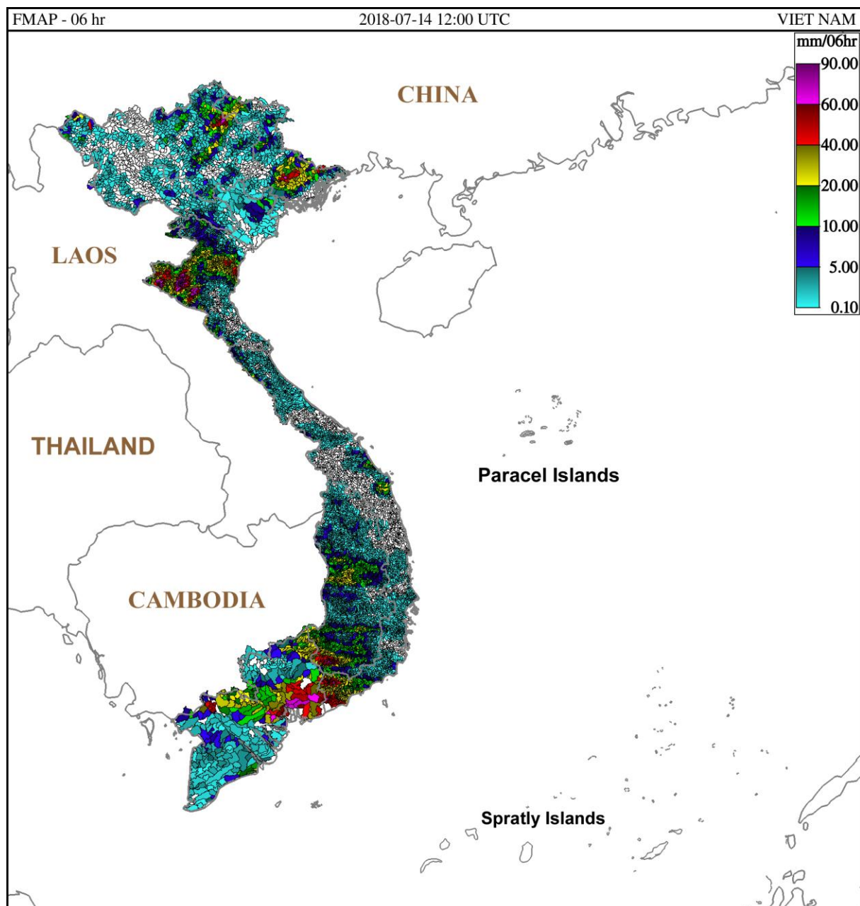
Hình 2: Dự báo lượng mưa trung bình lưu vực 6 giờ tính từ 19h ngày 14/07/2018 giờ địa phương
