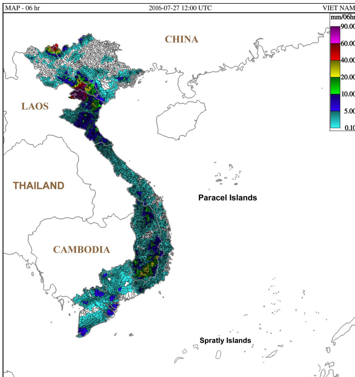
Hình 1. Lượng mưa lũy tích 6 giờ trung bình từng lưu vực tính đến 19h ngày 27/07/2016 giờ địa phương
