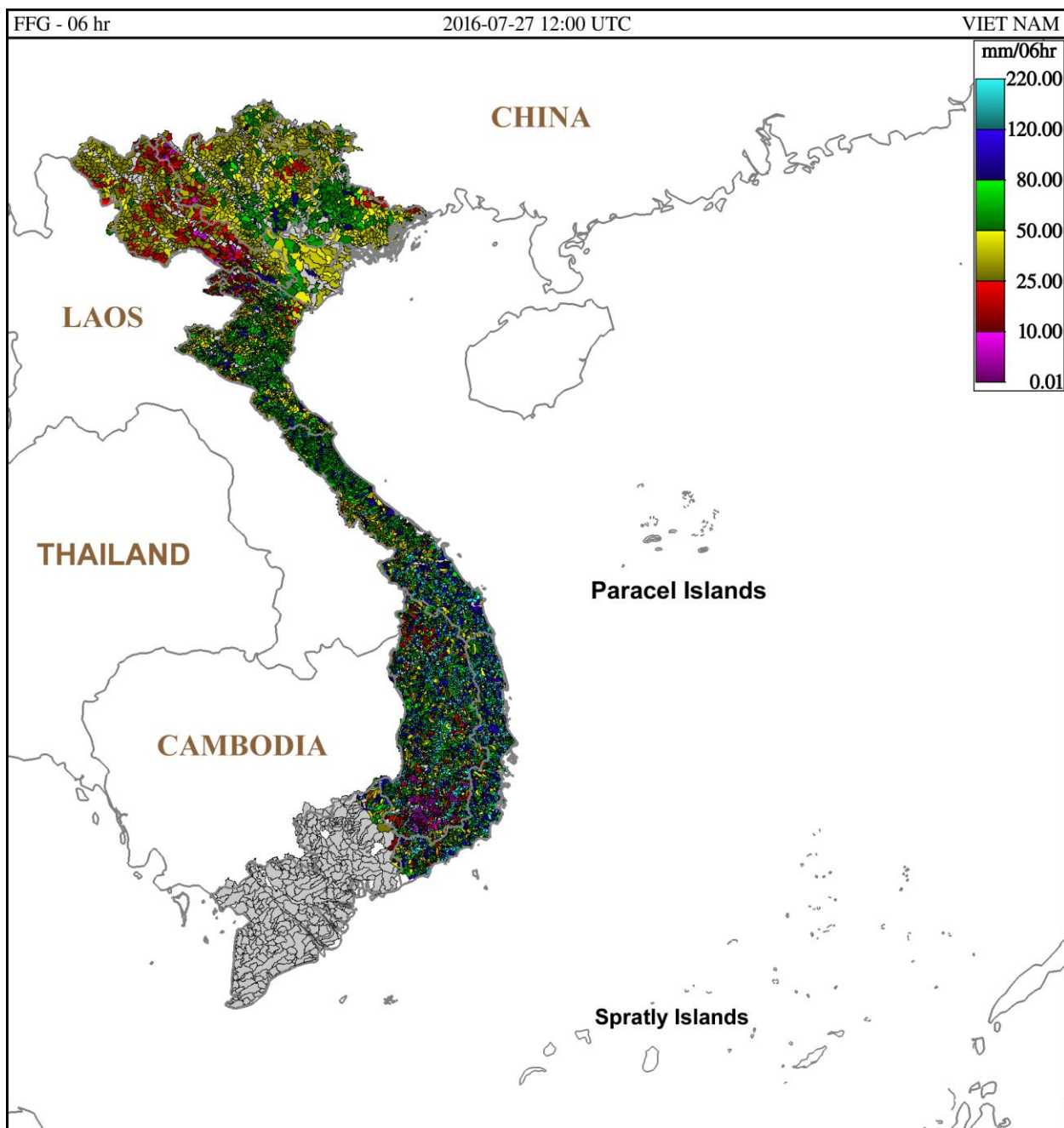
Hình 3: Ngưỡng mưa định hướng có khả năng sinh lũ quét trong 6 giờ tới tại các lưu vực từ 19h ngày 27/07/2016 giờ địa phương
