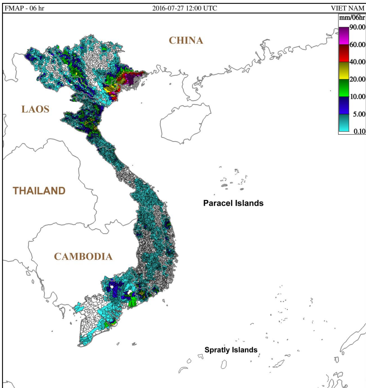
Hình 4: Dự báo lượng mưa trung bình lưu vực 6 giờ tính từ 19h ngày 27/07/2016 giờ địa phương
