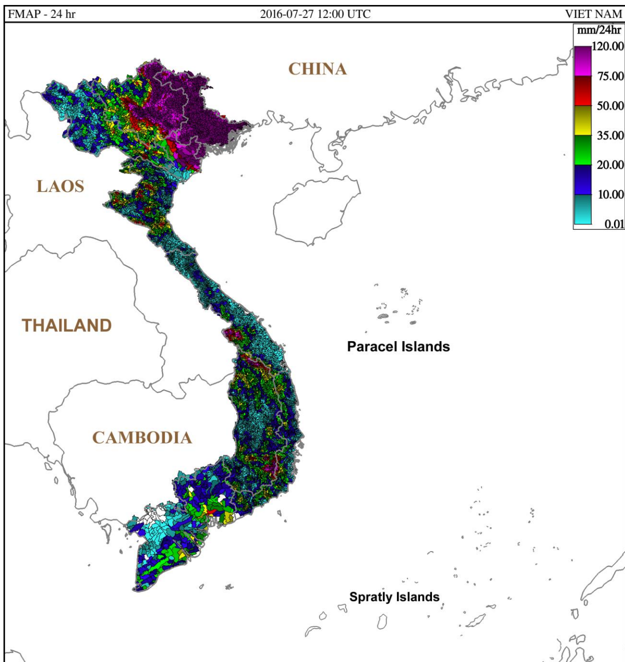
Hình 5: Dự báo lượng mưa 24h trung bình lưu vực tại thời điểm 19h ngày 27/07/2016 giờ địa phương
