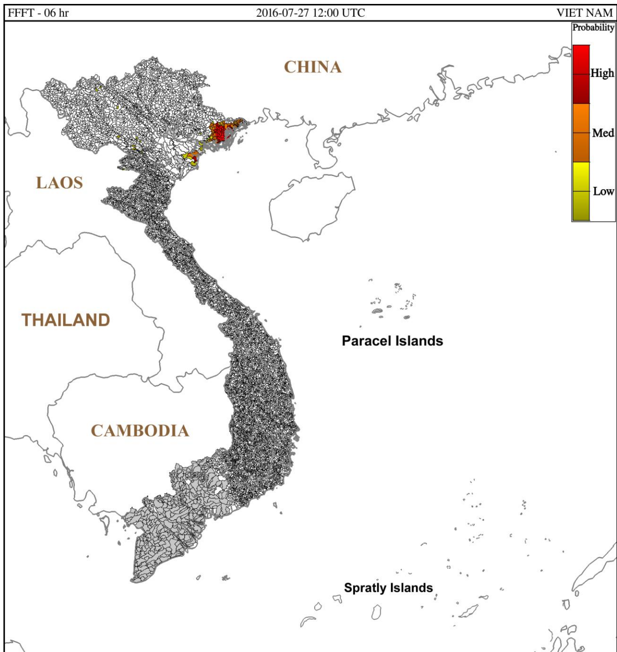
Hình 6: Nguy cơ lũ quét trong 6h tới tại tại thời điểm 19h ngày 27/07/2016 giờ địa phương
