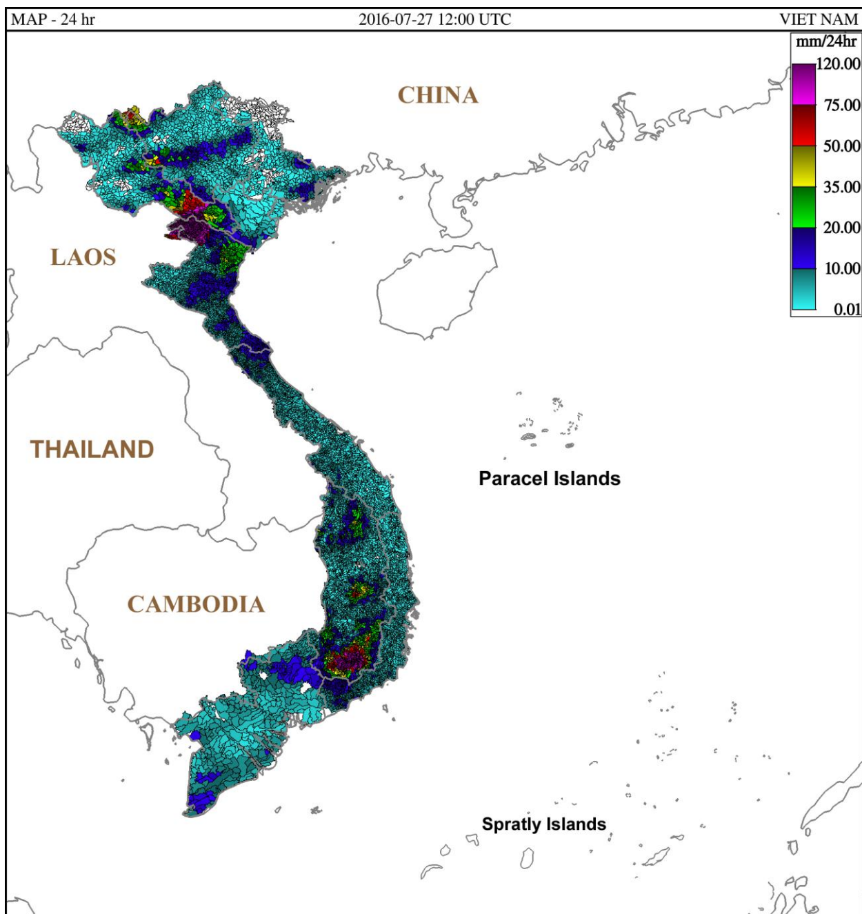
Hình 2. Lượng mưa lũy tích 24 giờ trung bình lưu vực tính đến 19h ngày 27/07/2016 giờ địa phương
